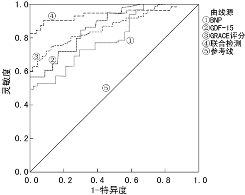
图 1 GRACE 评分、血清 BNP、GDF-15 诊断冠心病患者发生 HFrEF 的 ROC 曲线
